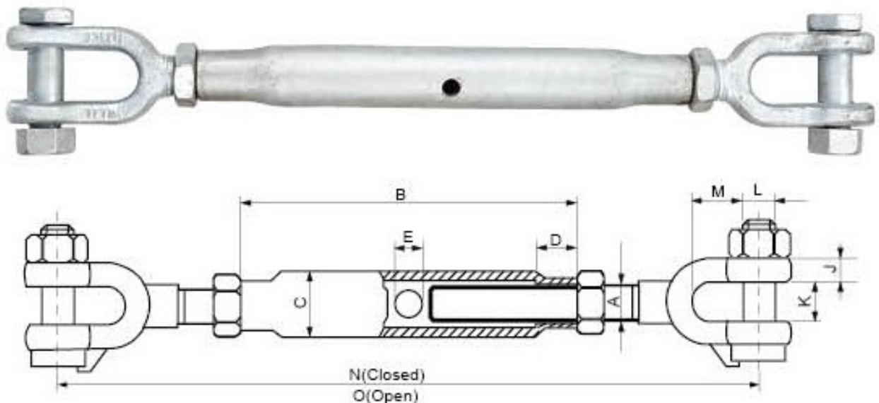
Рис.1 - Чертеж талрепа вилка-вилка (закрытого типа)
